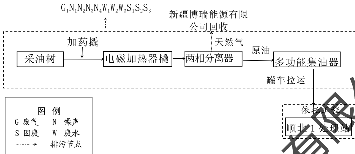
图 3.3-1 井场油气开采及集输工艺流程图
