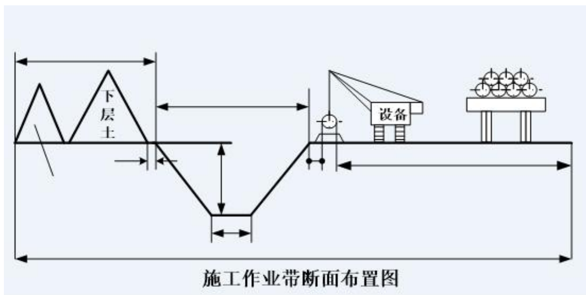
图 3.2-8 一般地段管道施工方式断面示意图
