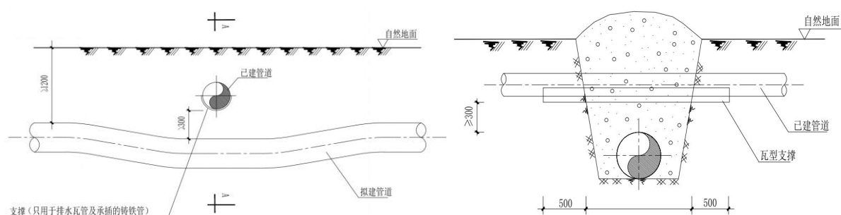
图 3.2-9 管道交叉施工作业示意图
