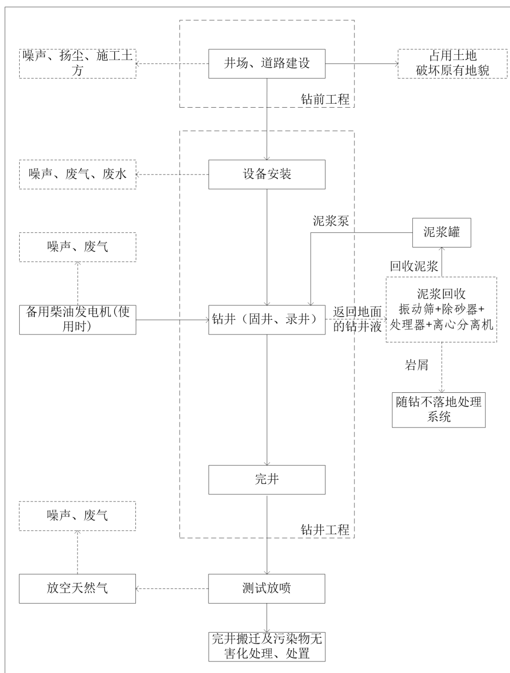
图 3.3-3 钻井工艺流程及污染物排放示意图
