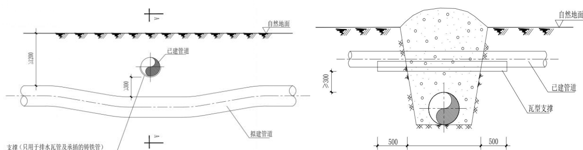
图 3.3-6 管道交叉施工作业示意图
