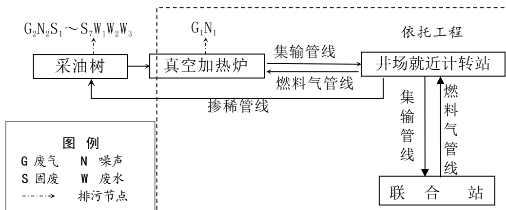
图 3.3-3 油气开采及集输工艺流程图
