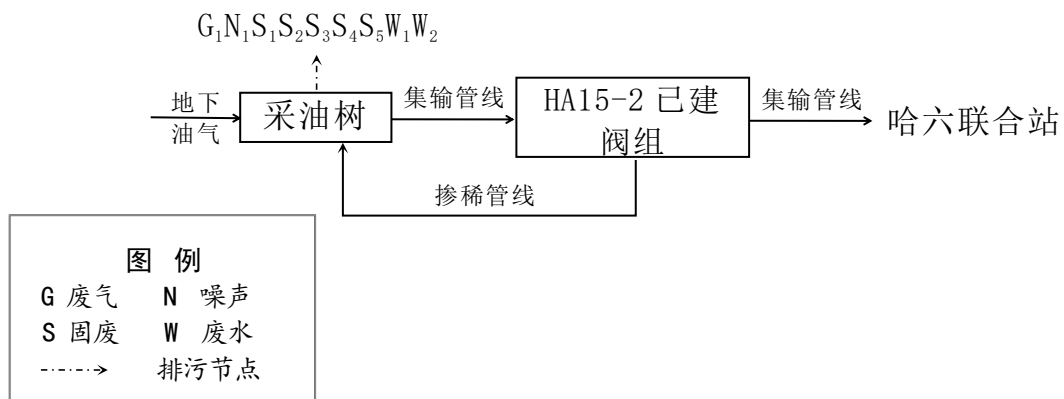
图 3.4-3 HA16-15X 井场油气开采及集输工艺流程图
