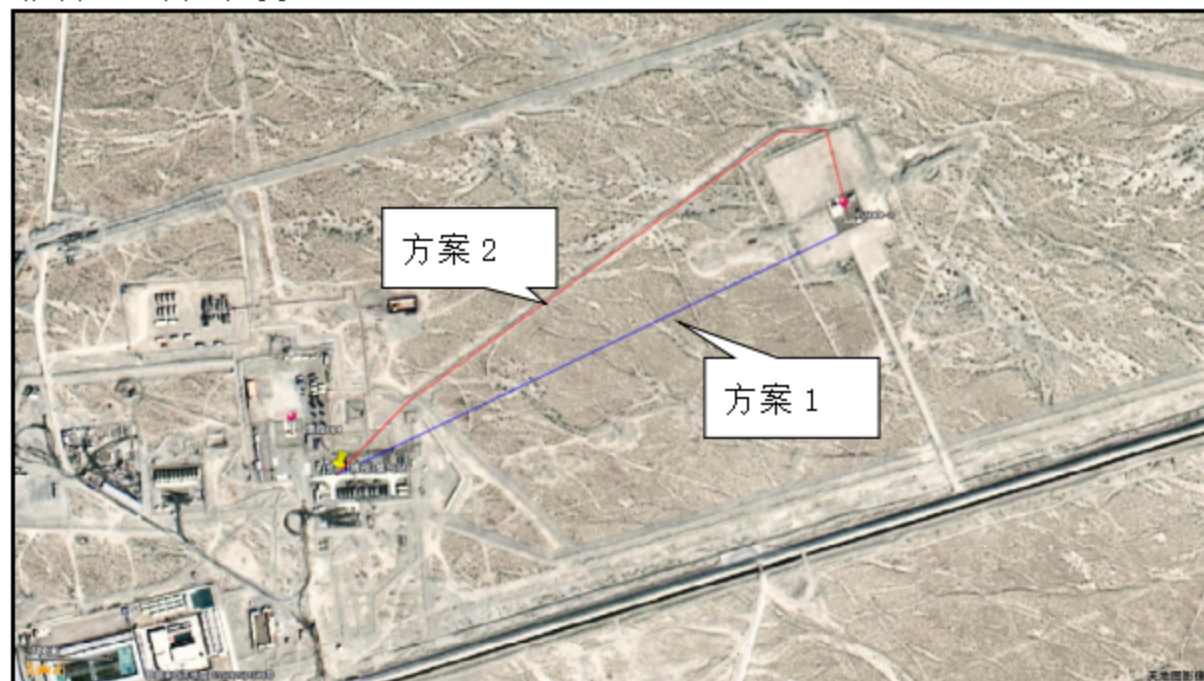
图 3.7-2 BZ104-2 排水管线线路比选方案示意图
