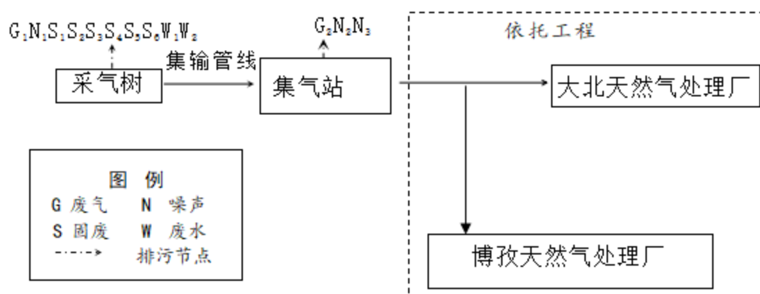
图 3.5-3 井场油气开采及集输工艺流程图
