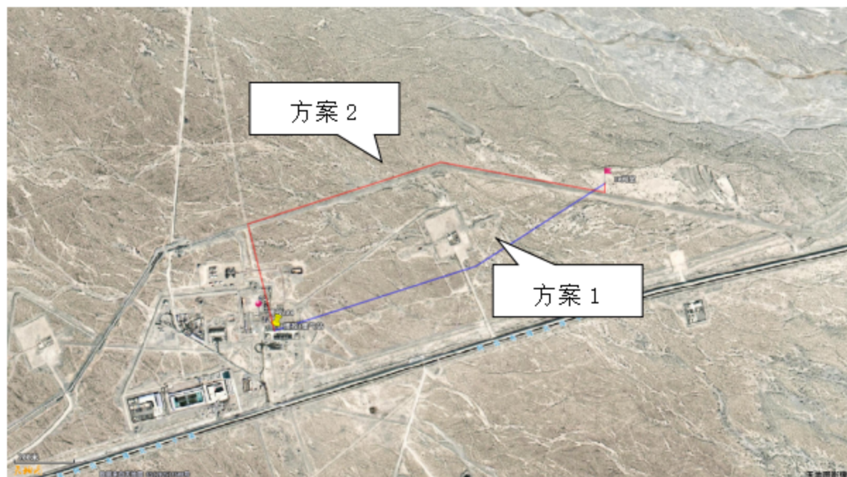
图 3.7-3 博孜 1 集气站排水管线线路比选方案示意图
