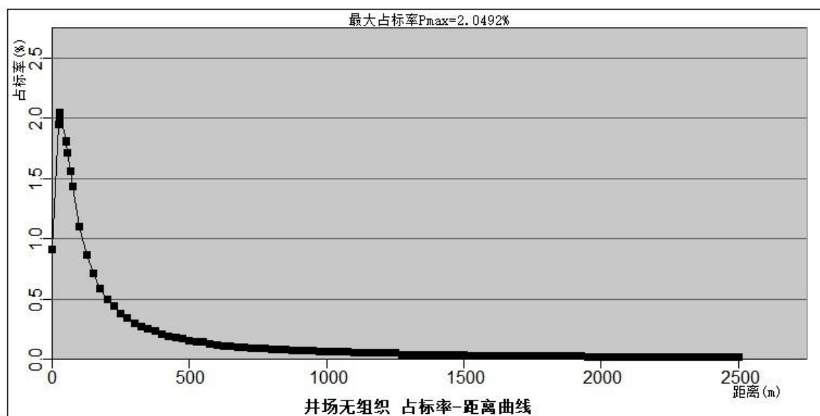
图 2.5-1 无组织废气占标率-距离曲线图
