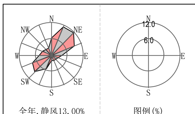
图 5.5-1 近 20 年风频玫瑰图
