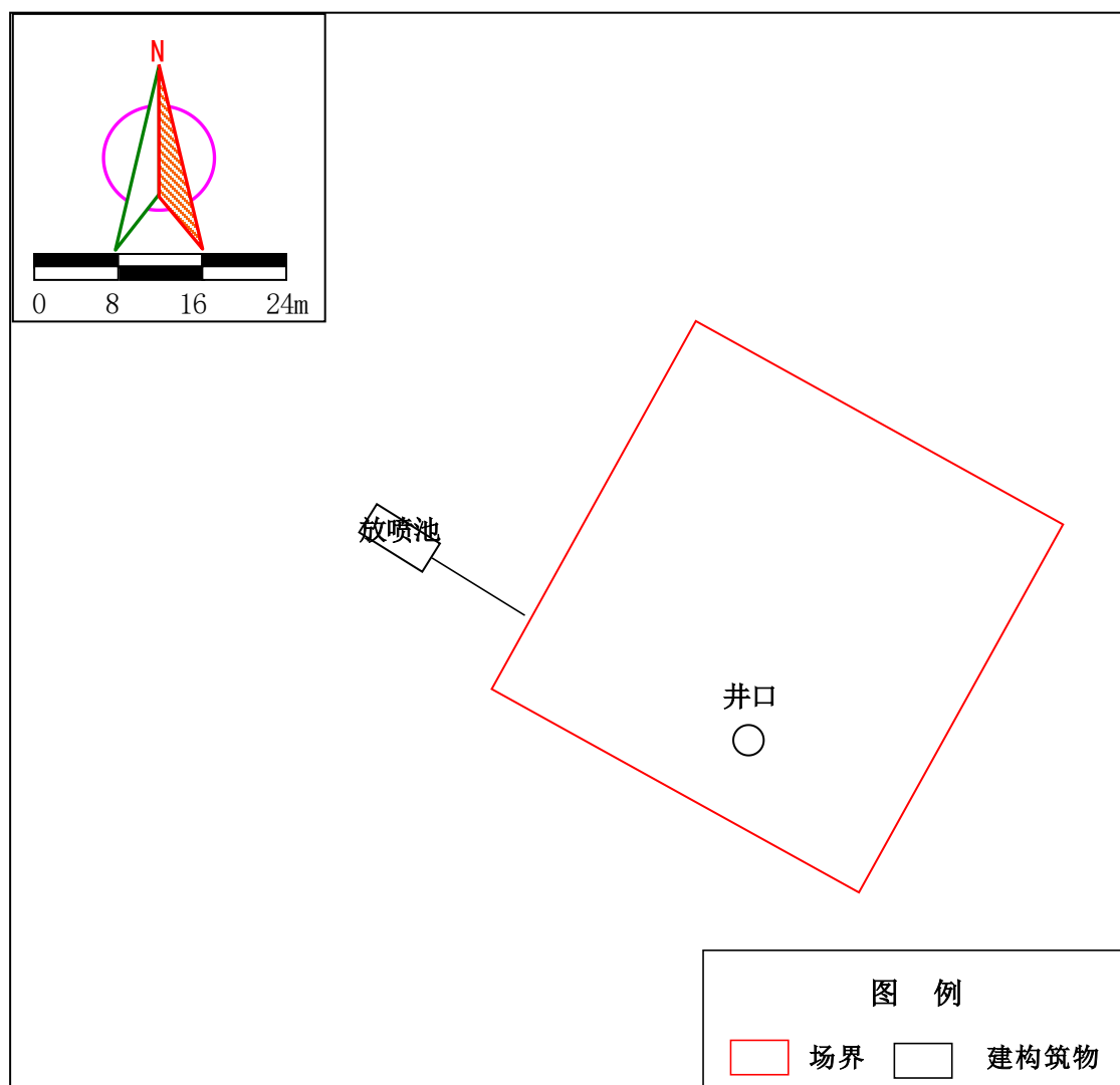
图 3.3-1 YueM21-H3 井场运营期平面布置示意图
