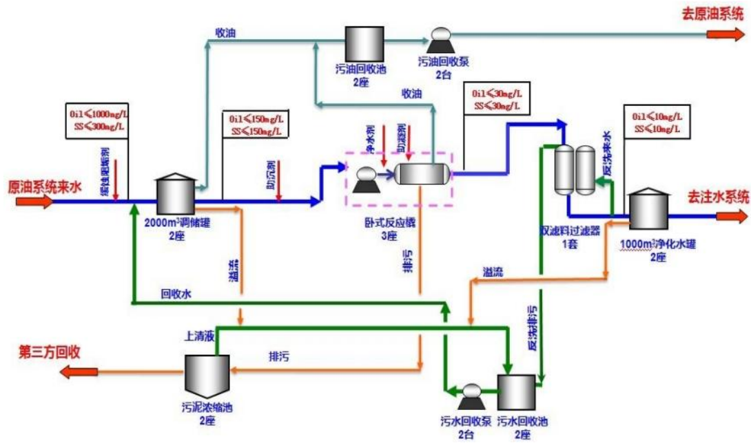
图 3.1-3 联合站水处理工艺流程图
