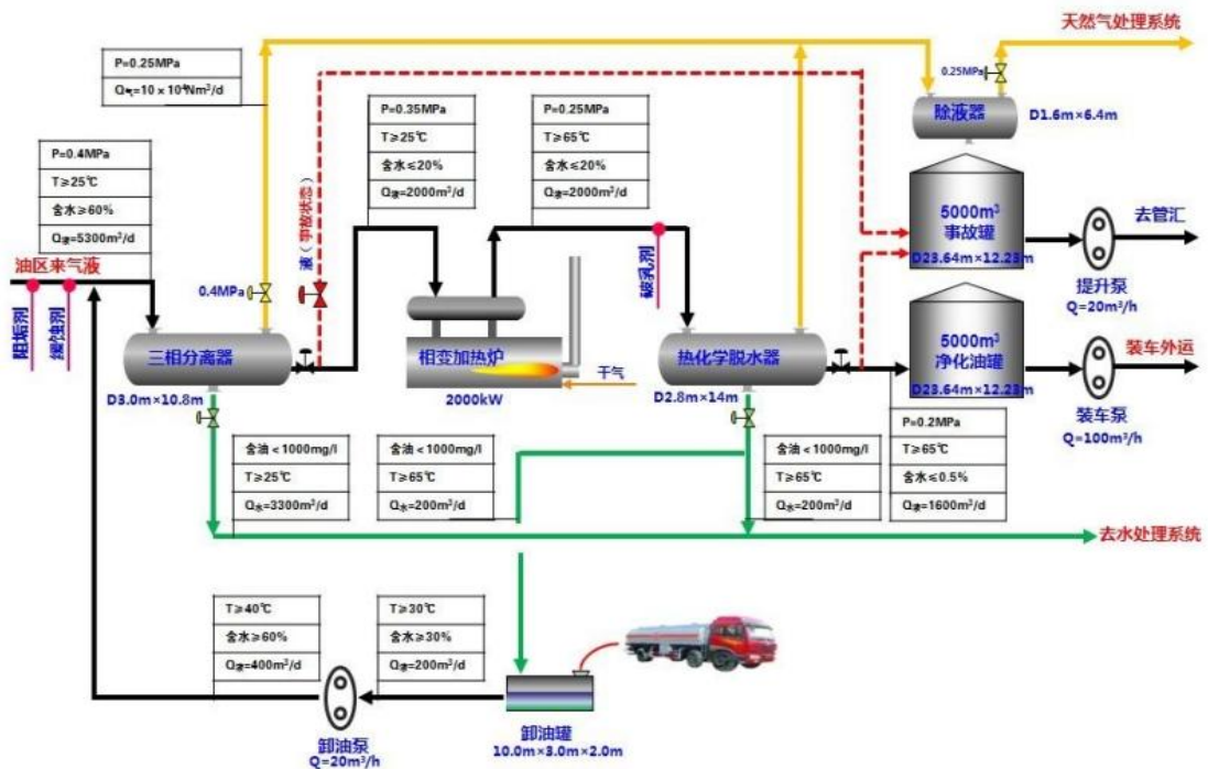
图 3.1-1 油气开采工艺流程图
